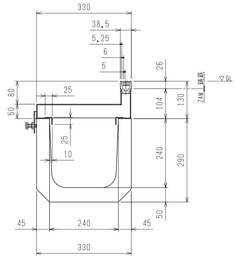
U字溝 240 600L
