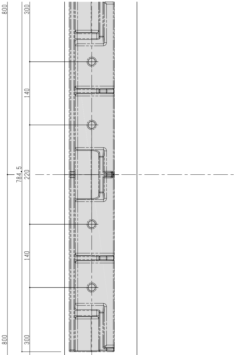
欠きこみ部拡大図 S:1/5 (A3)
