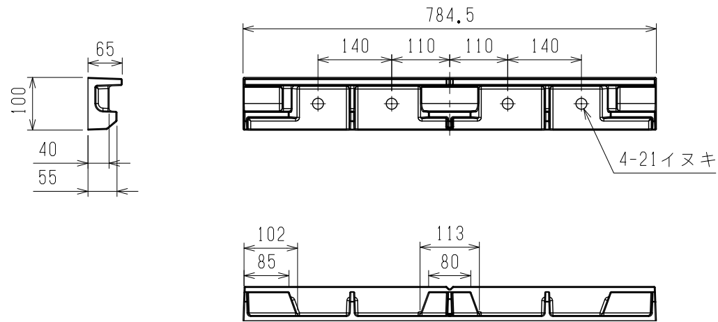
鑄鉄製 支持部材 (12kg/個)
