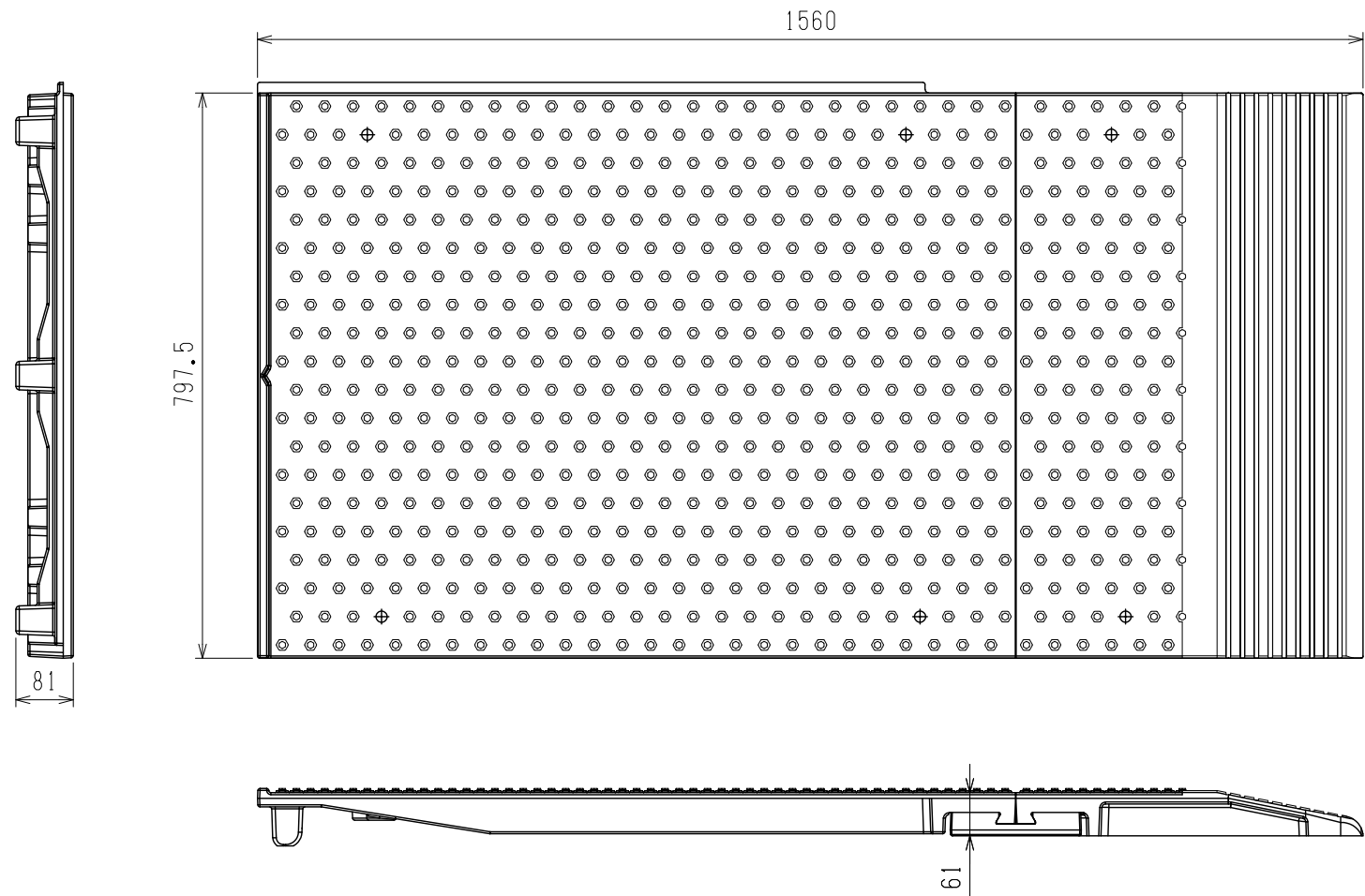
鑄鉄製 渡り板 (291kg/枚)
